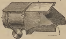
Fig. 204 Prisme disposé pour les projections verticales et de côté
