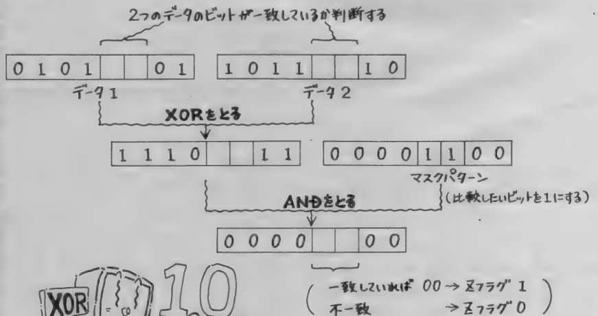
▶ 図6 XOR命令を使って、ビットの一致を確認する。
