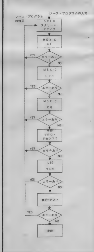
図1 MSX-Cのプログラム開発手順
