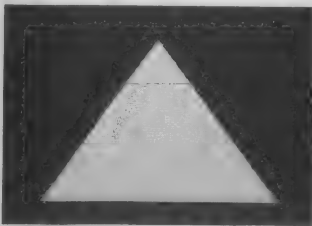
◆最初に正三角形を描き、それぞれの3辺を結び正三角形をくり抜いていく。
