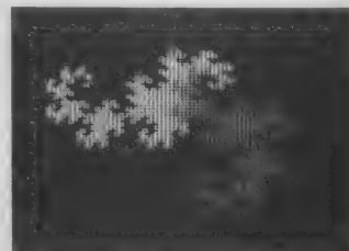
▲ただの線なのに、平面を埋めつくしてしまう、なまいきなドラゴンカーブだ。
