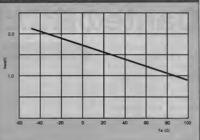
■ グラフ1 S8100の電気特性
