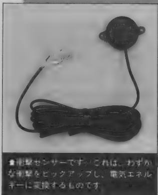
●小型精密センサーです。これは結露とともに抵抗値が急増に増加するもので、小型でどこでも取り付け可能です。
